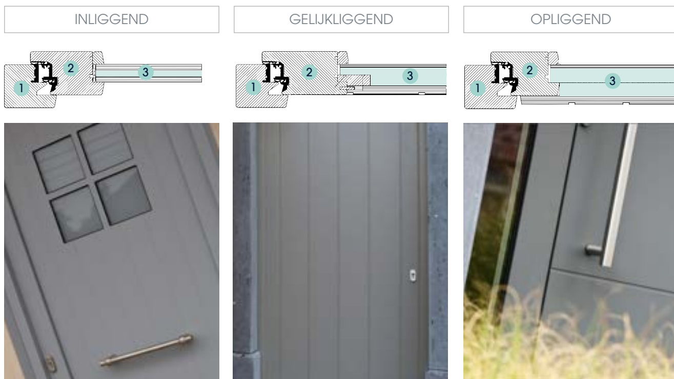
1 Kader 2 Vleugel 3 Vulling (paneel of glas)
